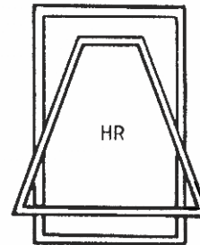
Kiểu mở lật theo trụ ngang đảo
