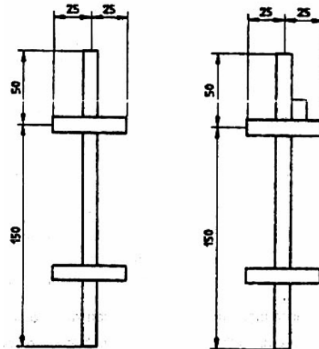
Hình 2 - Mẫu thử
